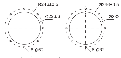
* หน่วย : mm. *
