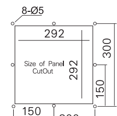
* หน่วย : mm. *
