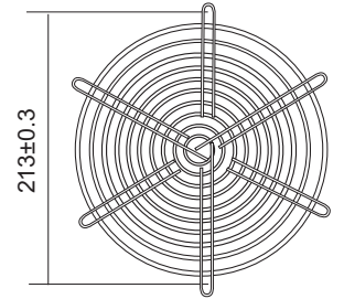
* หน่วย : mm. *
