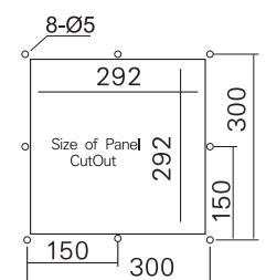
* หน่วย : mm. *
