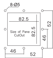
* หน่วย : mm. *
