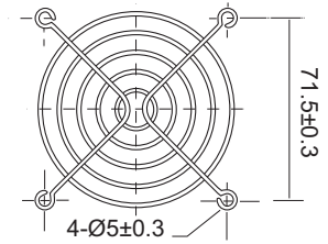
* หน่วย : mm. *
