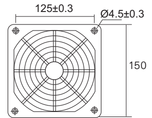
* หน่วย : mm. *
