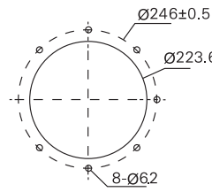
* หน่วย : mm. *
