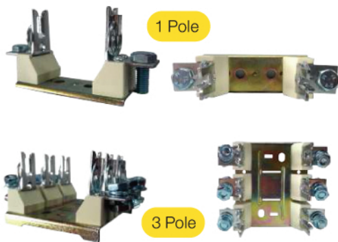
ฐานพิวส์ใบมิด รุ่น HRC-FUSE BASE NH (Size 00,1,2)
